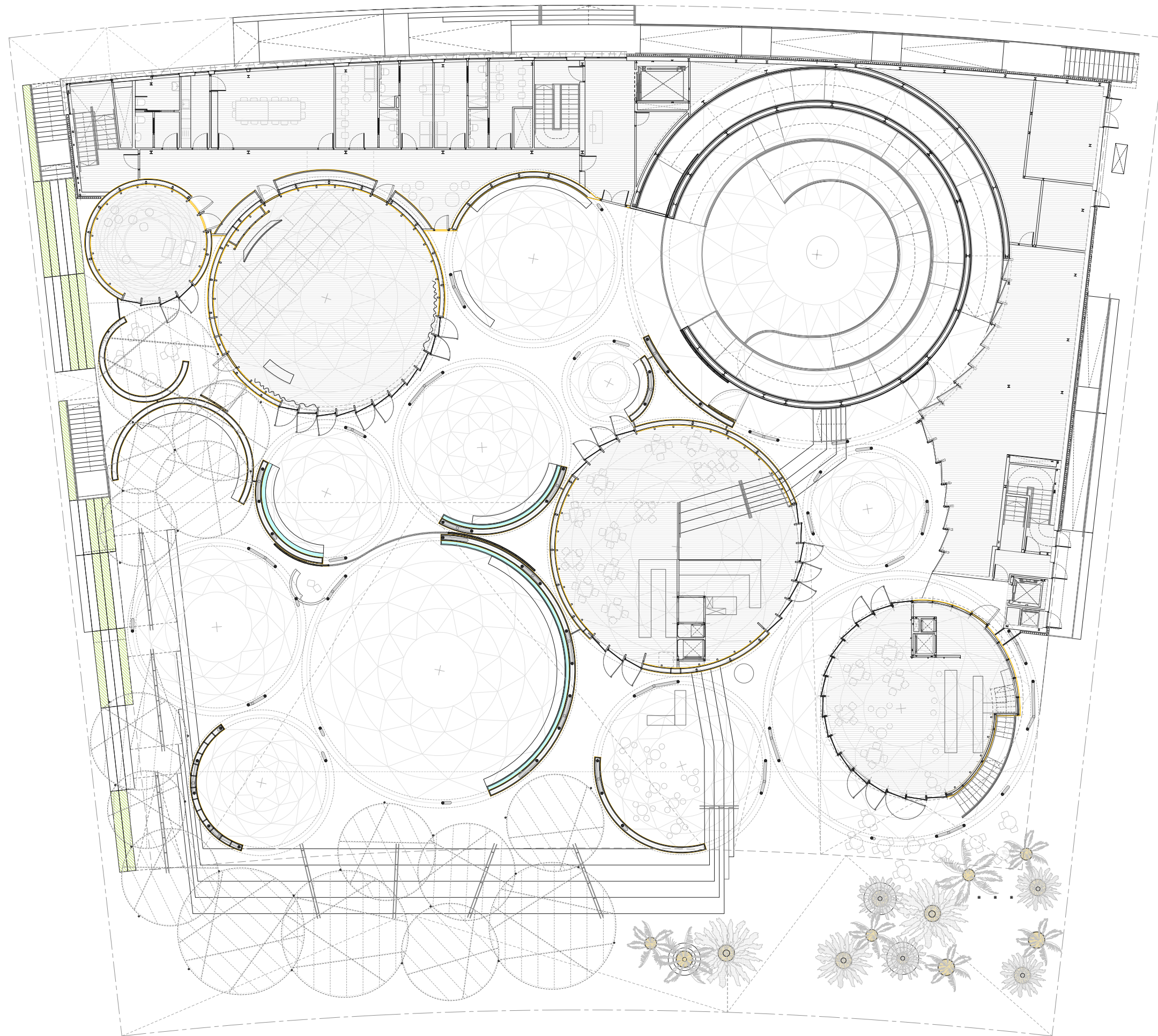
PLANTA BAJA-ACCESO
