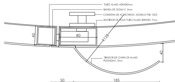
TIRADOR 2 E 1:5
