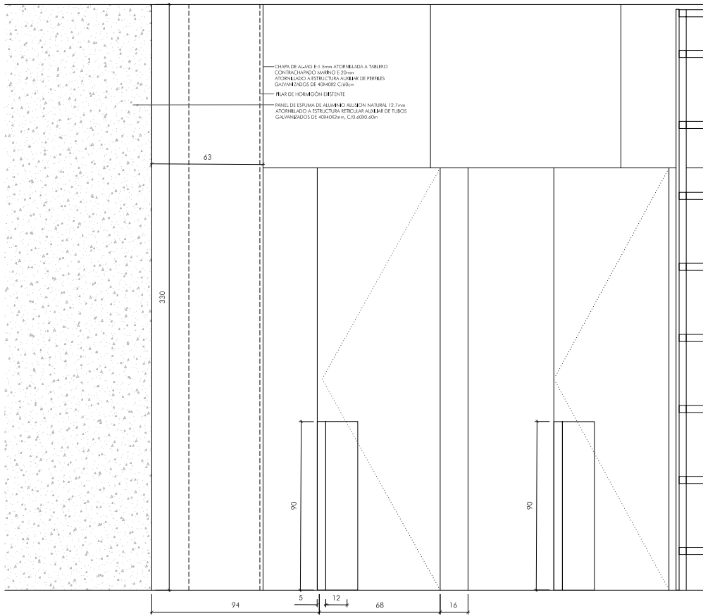
ALZADO E 1:30
