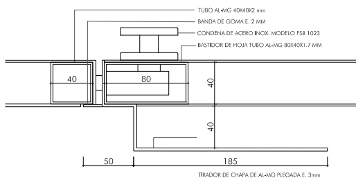
TIRADOR 1 E 1:5
