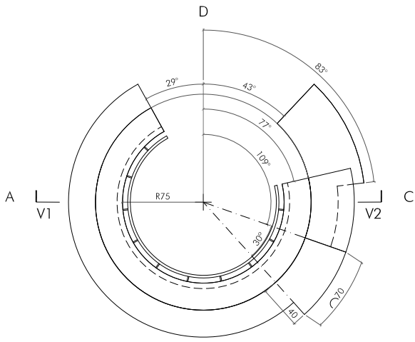
PLANTA 1:50
