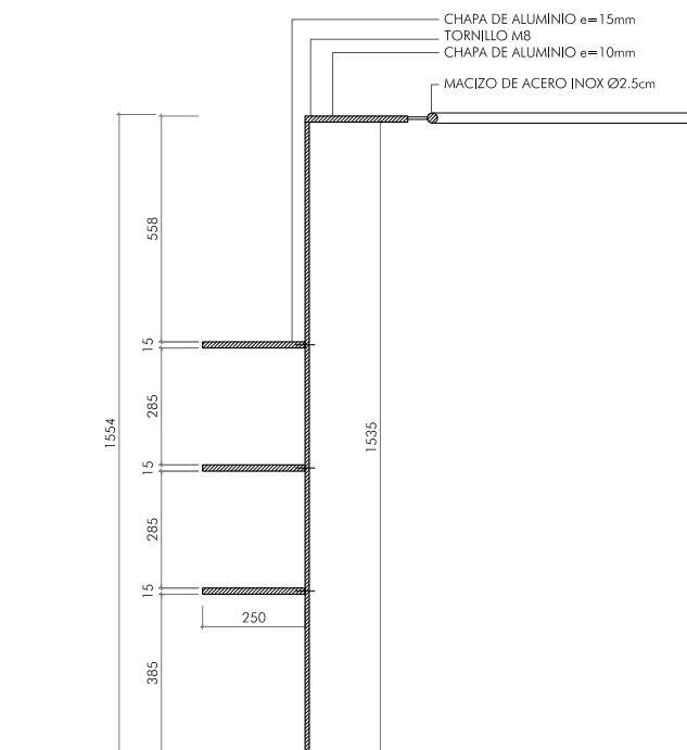
SECCIÓN V1 E 1:20
