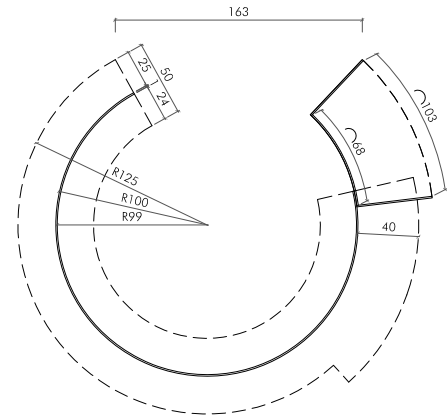
SECCIÓN H1 E1:50
