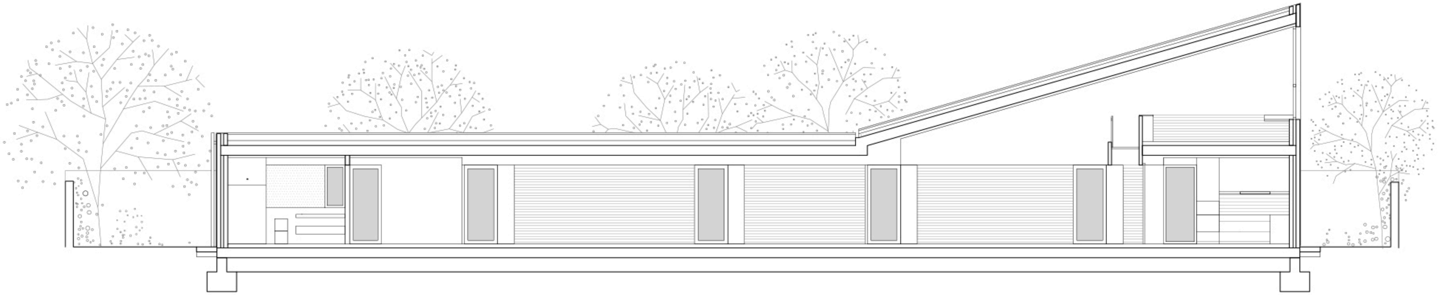
SECC LONGITUDINAL 2
