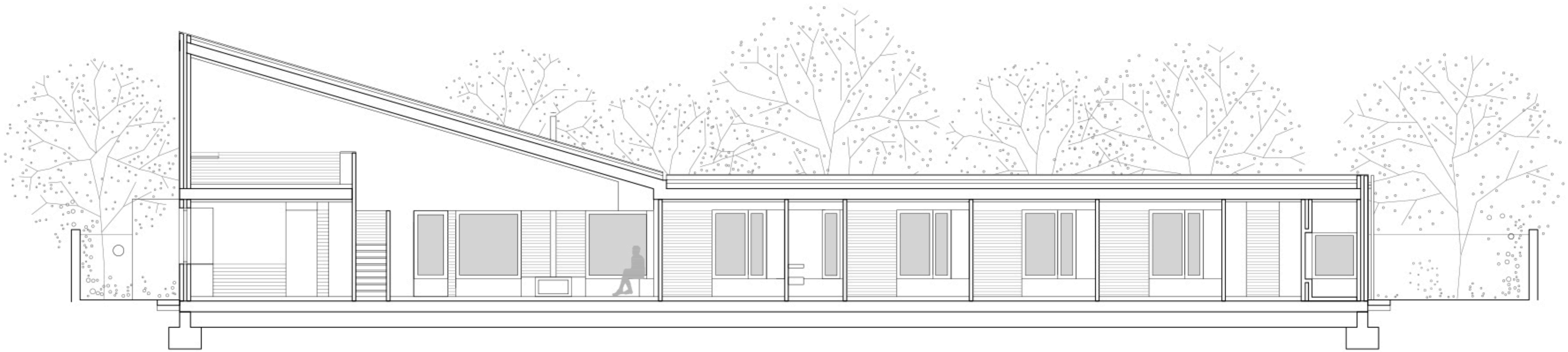
SECC LONGITUDINAL 1
