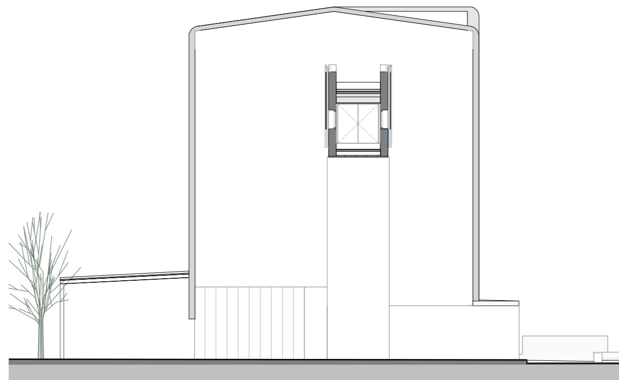
ALZADO OESTE
