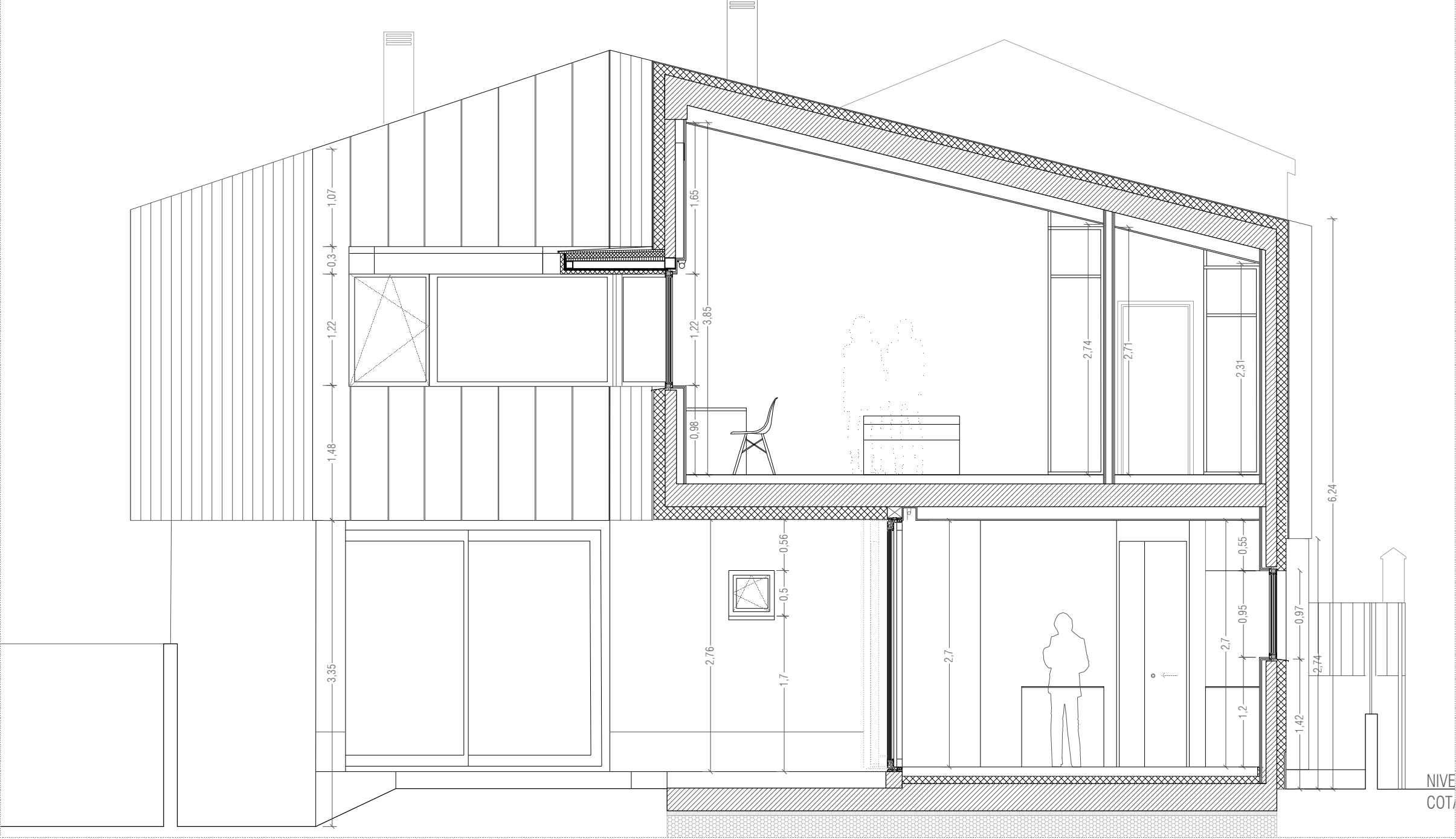
SECCIÓN TRANSVERSAL
