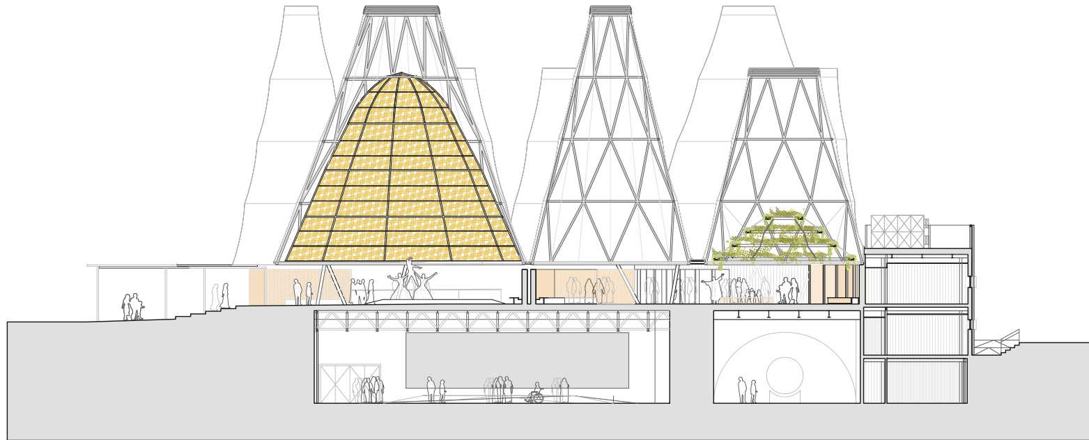
SECCIÓN BB'
