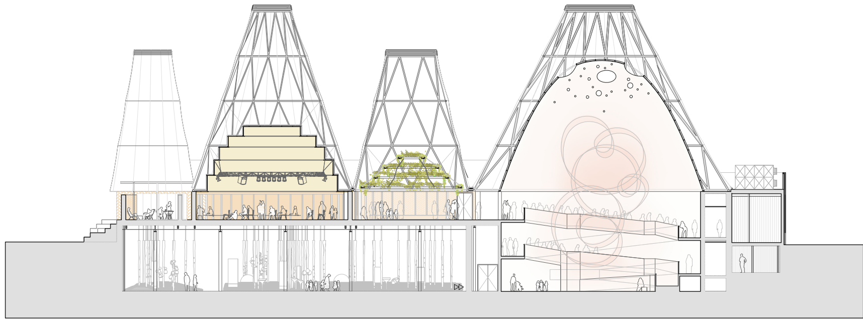
SECCIÓN DD'
