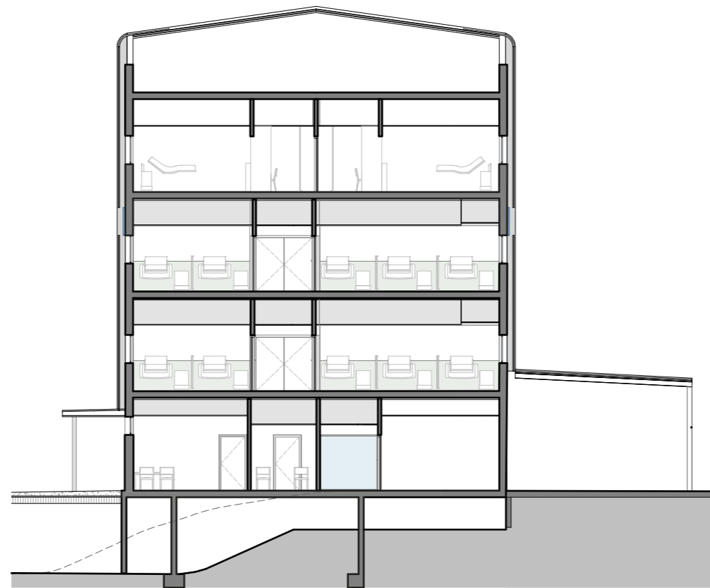
SECCIÓN TRANSVERSAL
