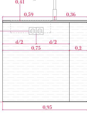
Alzado 3-3´
