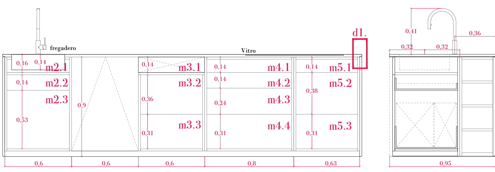
Alzado exterior 1-1´
