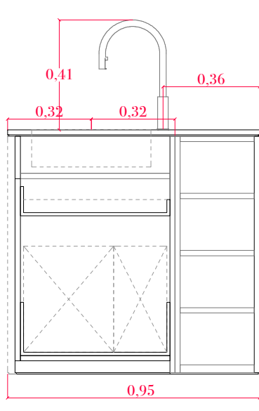
Alzado 3-3´
