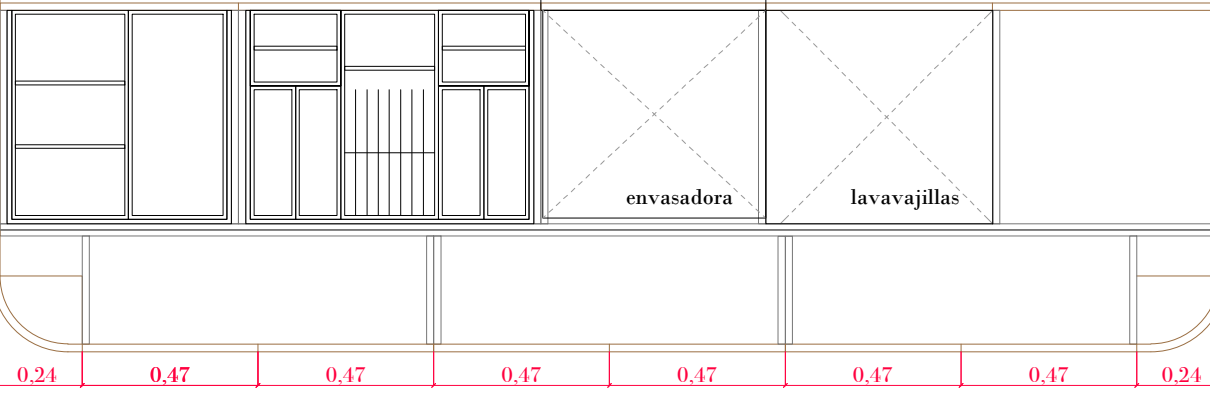
Planta seccionada
