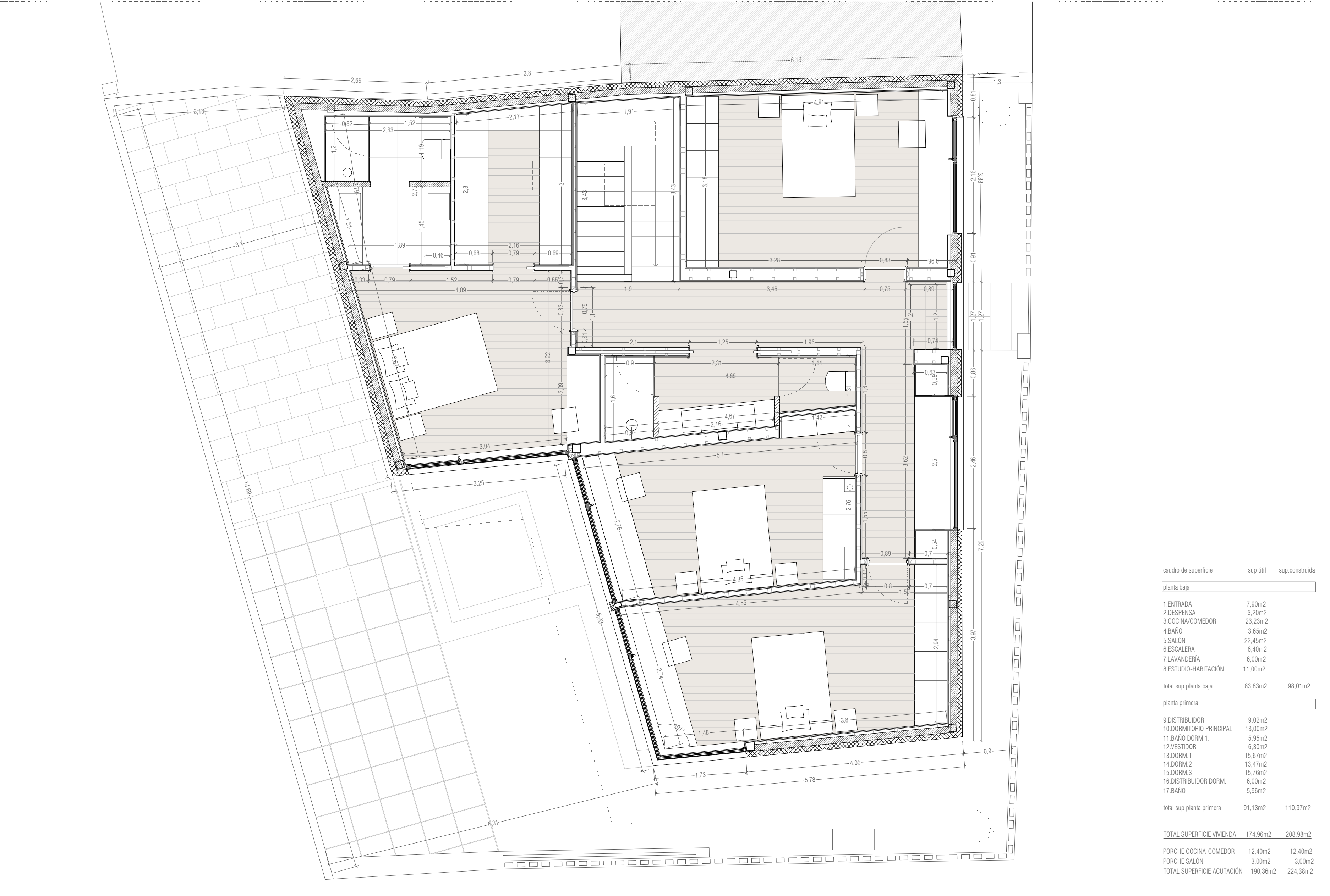
PLANTA PRIMERA
