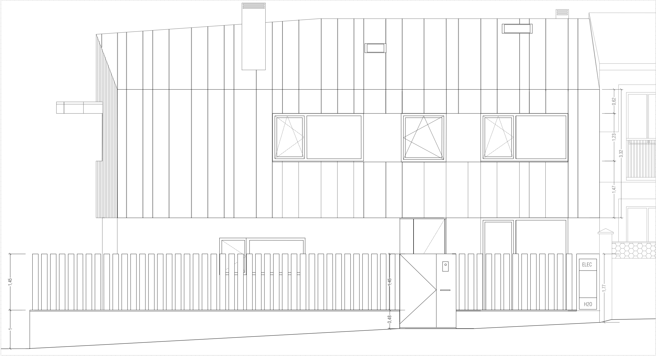
ALZADO CALLE MADRESELVA (EXT)
