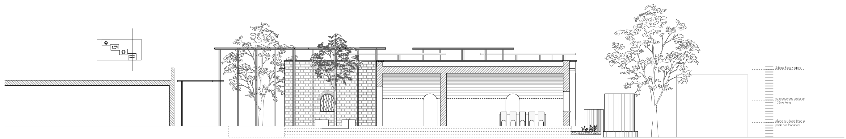
COUPE TRANSVERSALE 01
