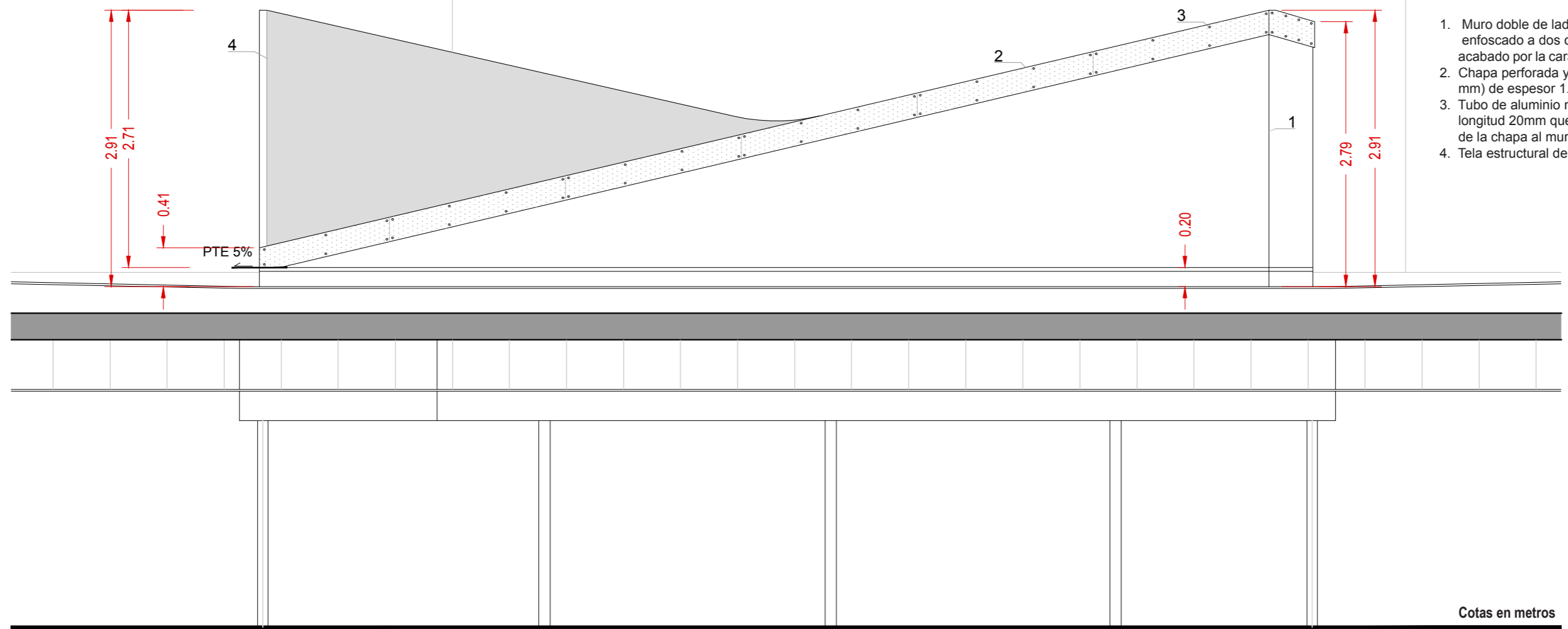
ALZADO ESTE
