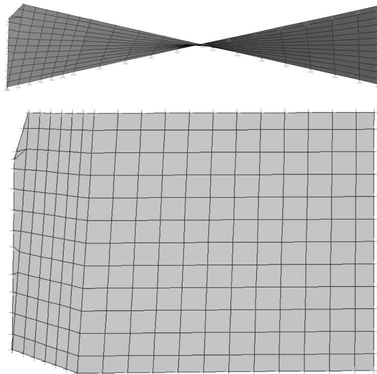
Planta y alzado de la cubierta (Paraboloide hiperbólico) en el modelo de cálculo.
