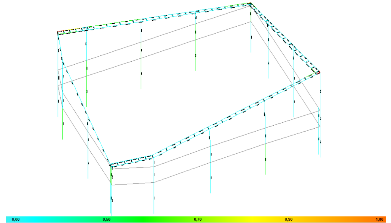
Resultado de la comprobación de los perfiles metálicos de la nueva estructura.
