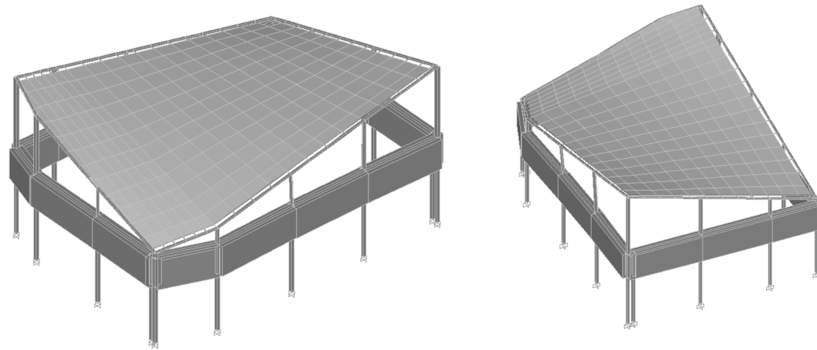
Geometría de la estructura de cubierta, junto con la original procedente de la modelización
