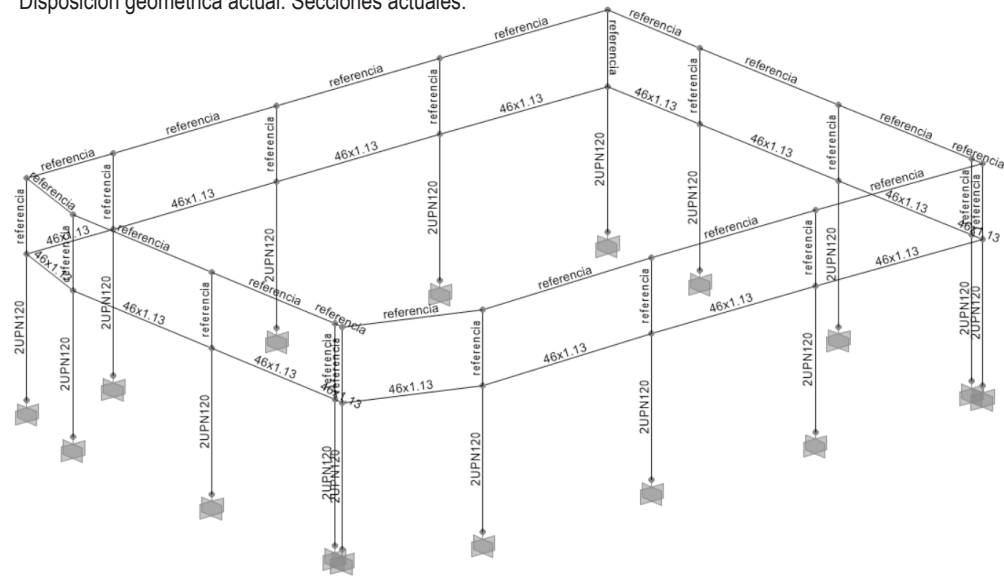
Disposición geométrica actual. Secciones actuales.
