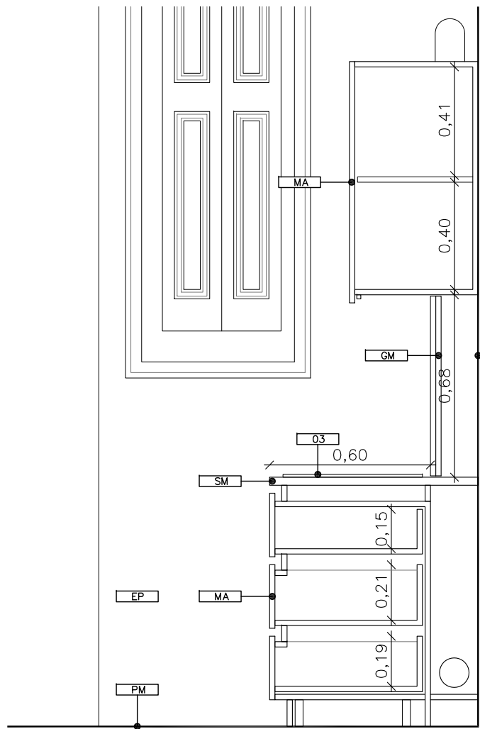
CUINA SECCIÓ B
