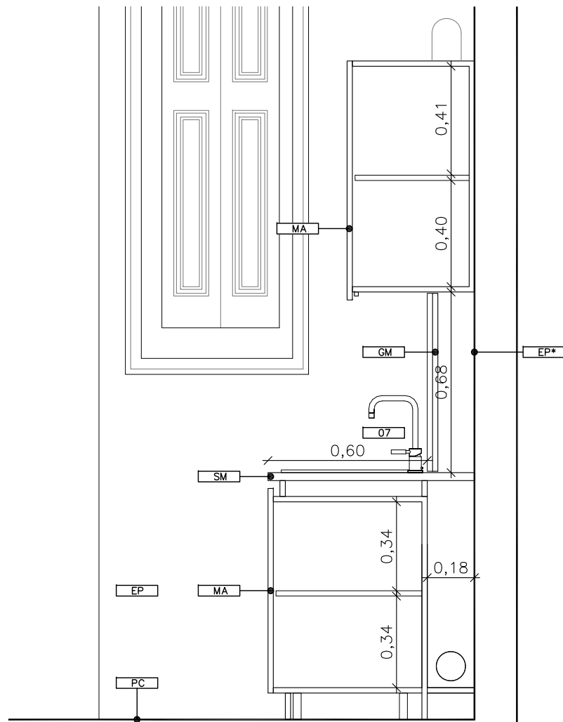
CUINA SECCIÓ C
