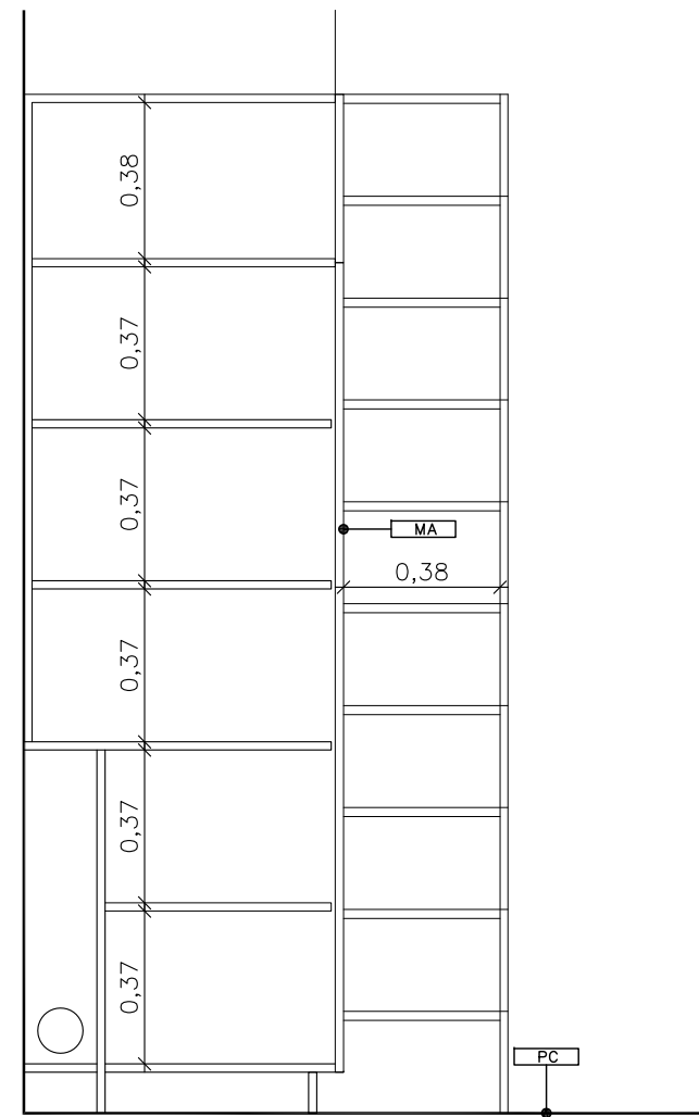
CUINA SECCIÓ D
