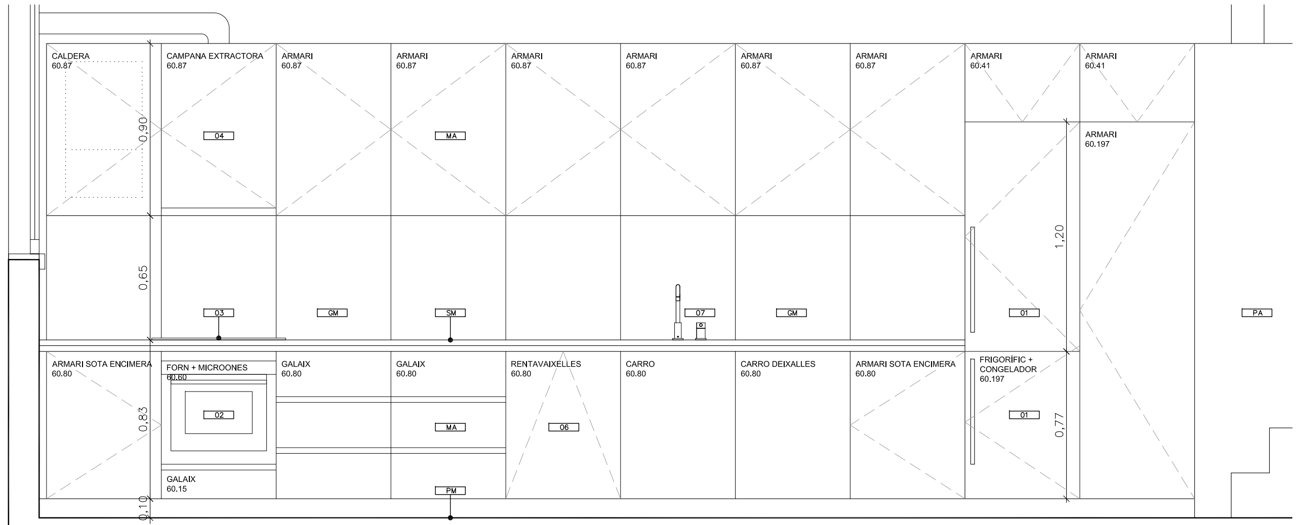
CUINA SECCIÓ A
