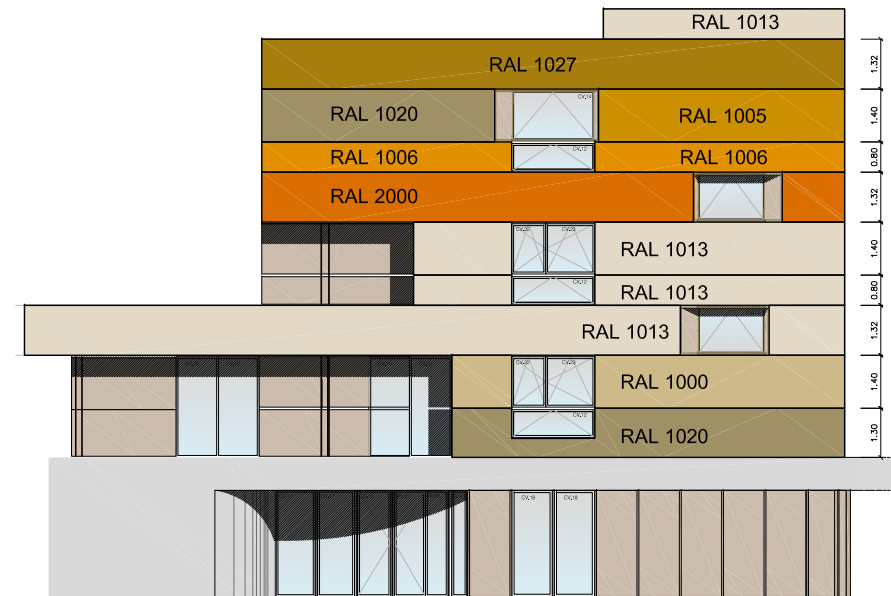
FACHADA CALLE. ALZADO SURESTE
