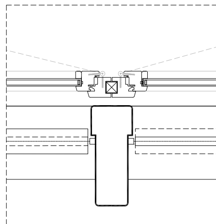
DETALL MUNTANT PREFABRICAT FAÇANA
