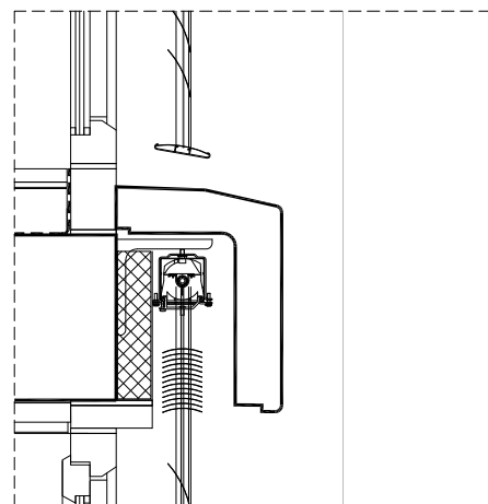
DETALL CANTELL DE FORJAT PREFABRICAT
