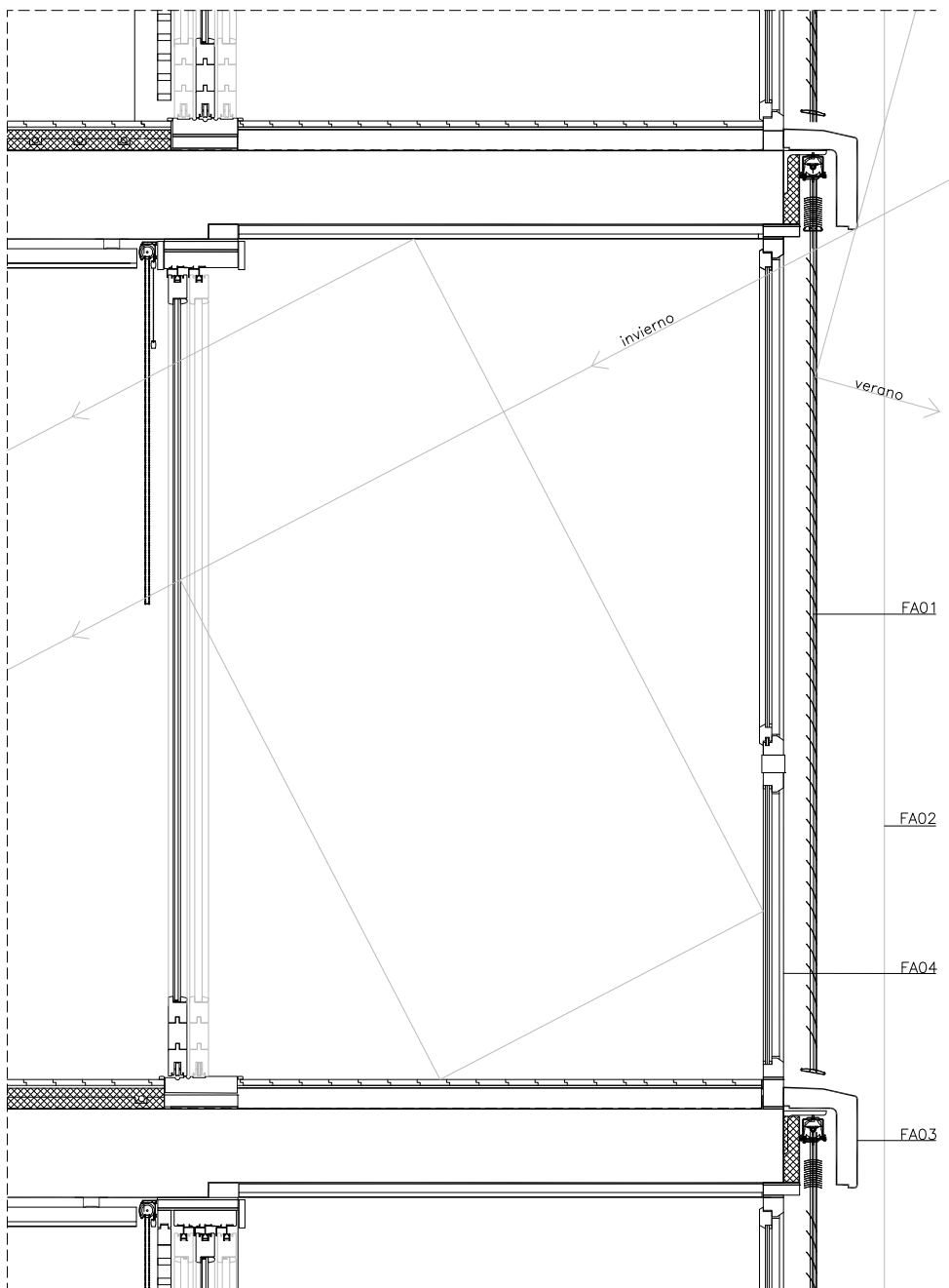
SECCIO COIXÍ CLIMÀTIC
