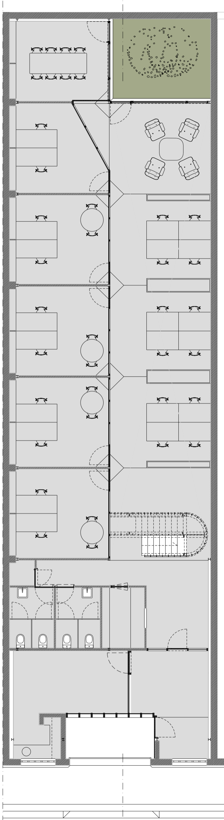
A. PLANTA DO PISO 0
