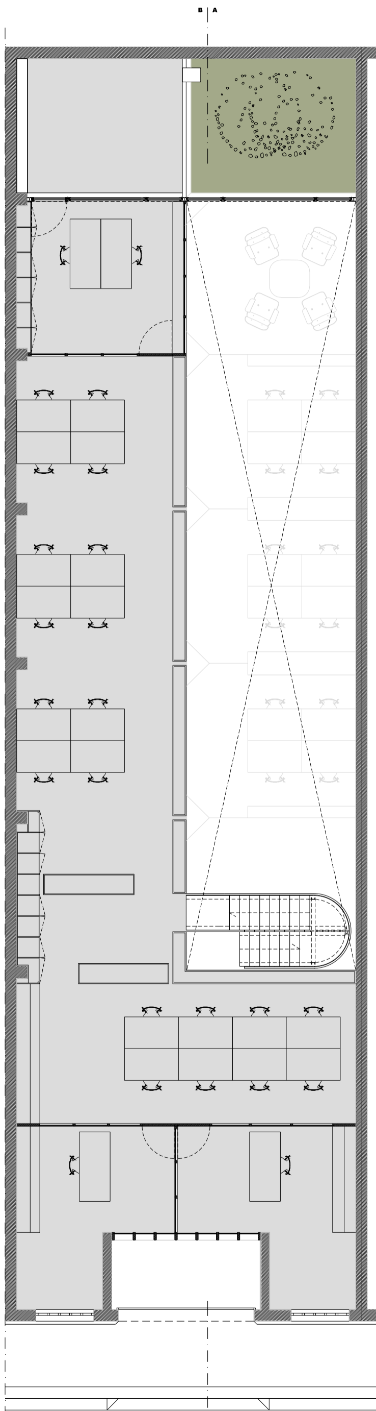
B. PLANTA DO MEZANINO
