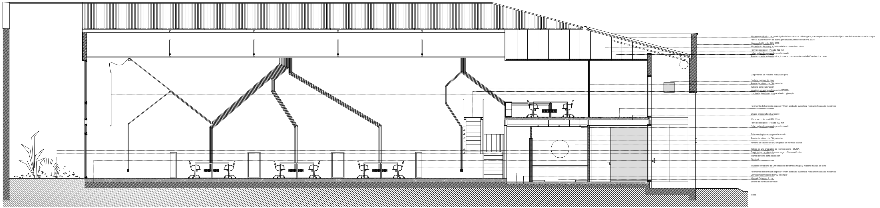
A. Sección LONGITUDINAL
