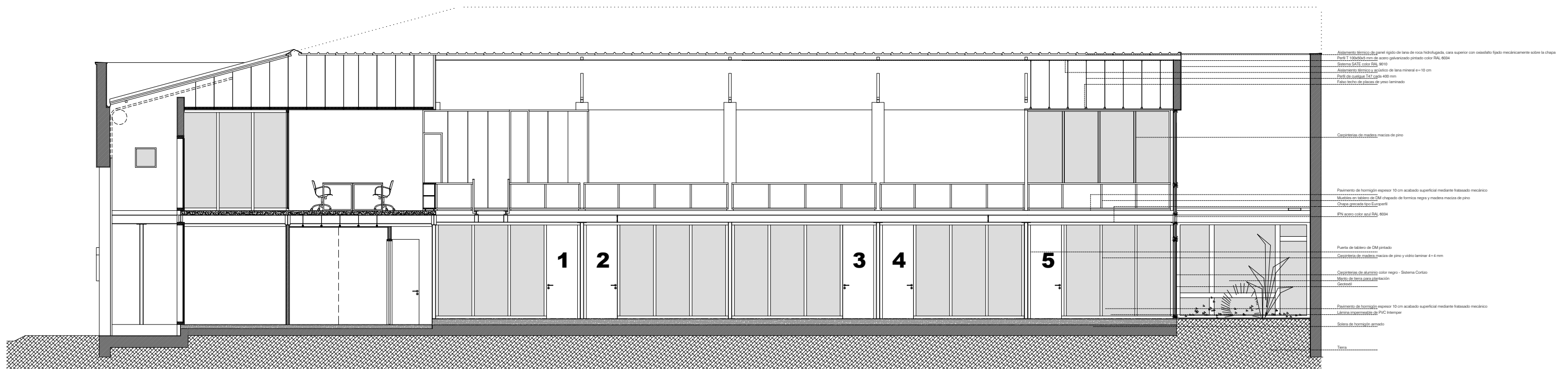
B. Sección LONGITUDINAL
