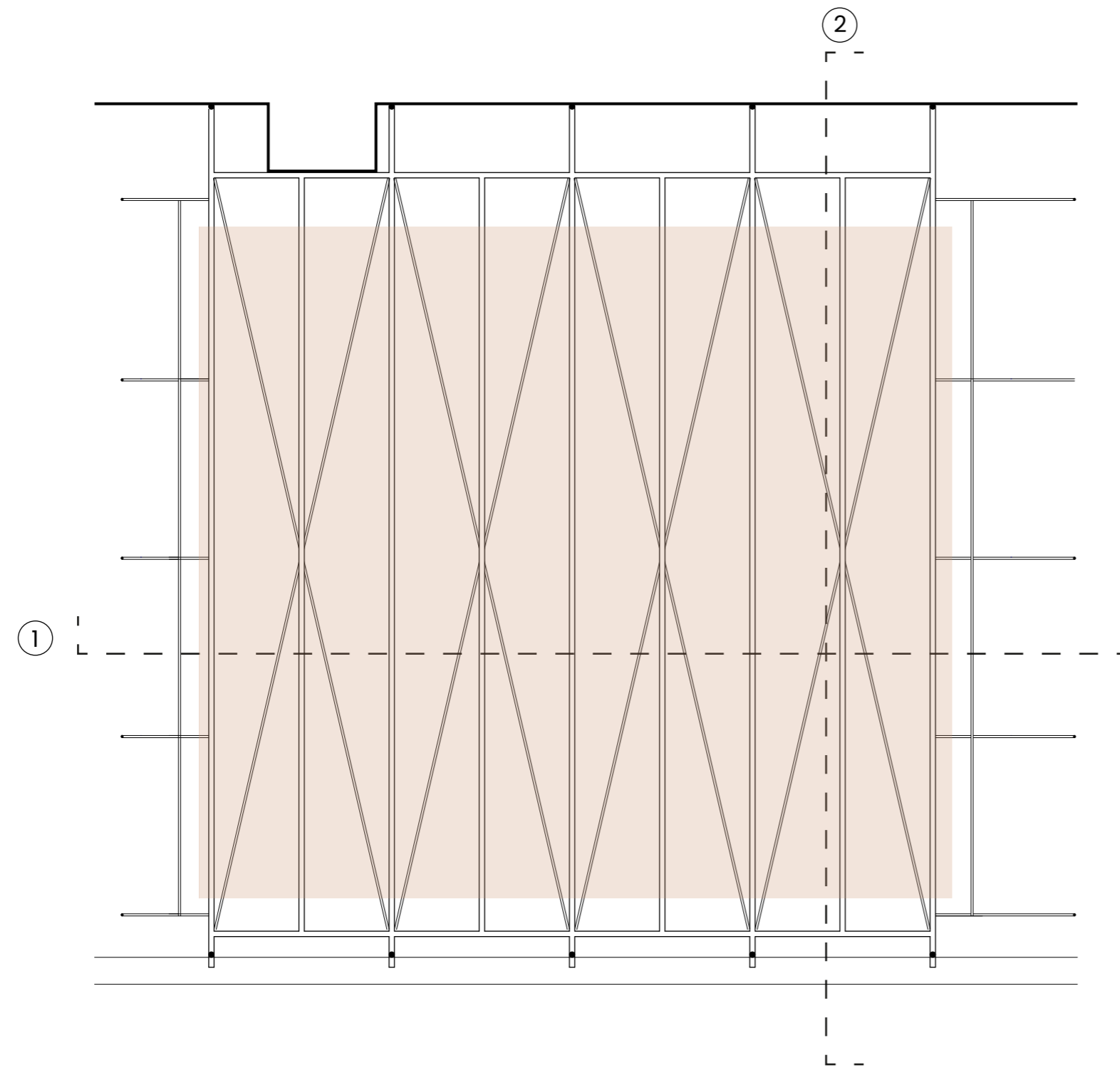
DETALLE ESTRUCTURA ALTILLO. ESCALA 1:20
