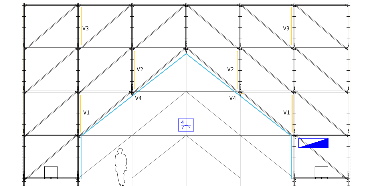
Sección interior BB
