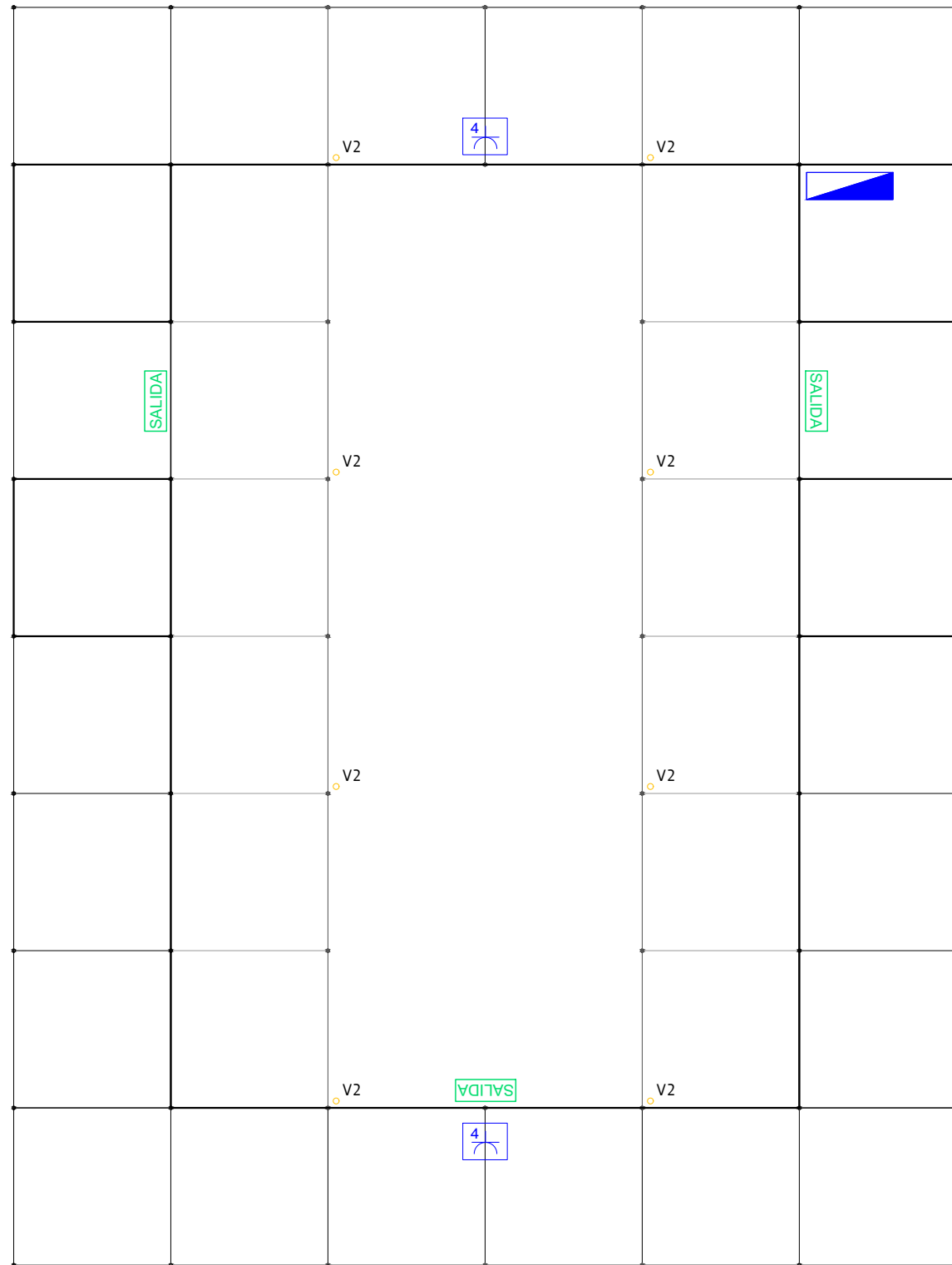
Planta nivel 2
