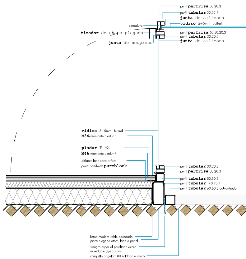
planta carpintería cocina
