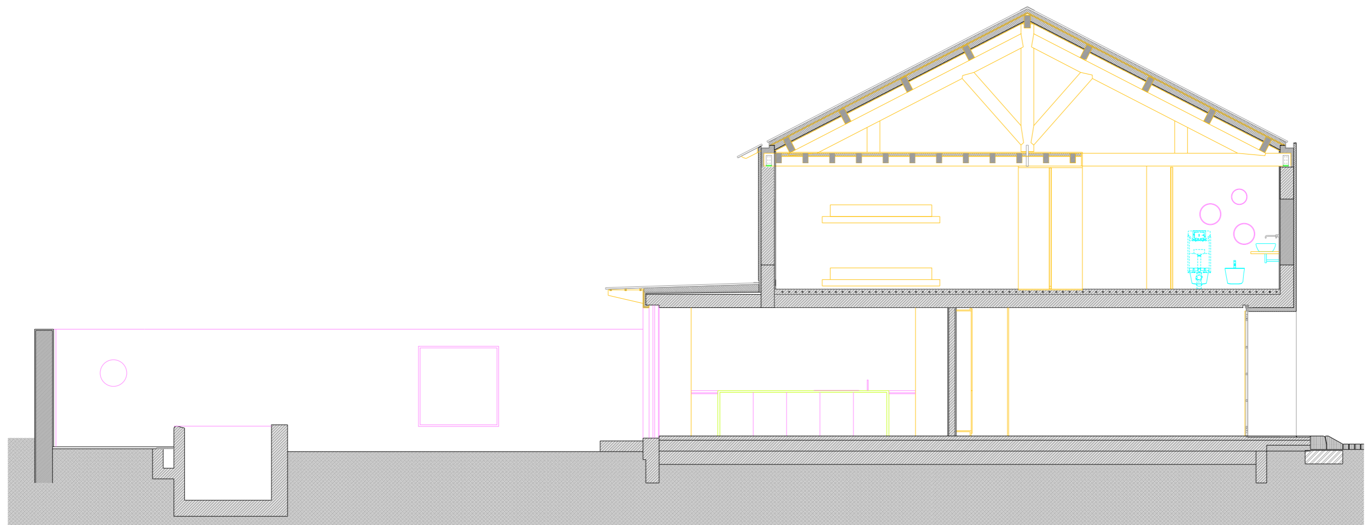
Longitudinal Section 3
