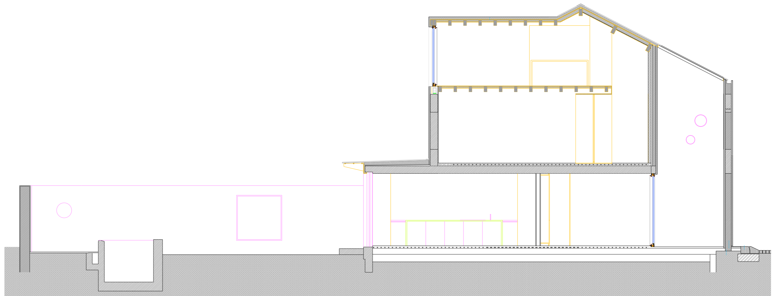
Longitudinal Section2
