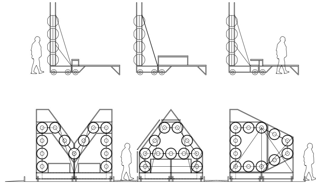
Alzados
