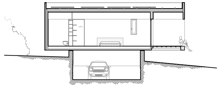
Sección C
