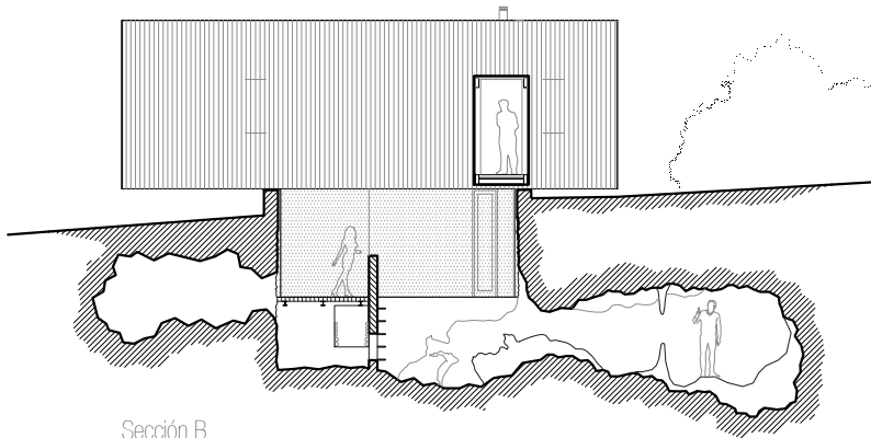
Sección B
