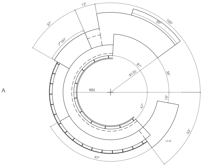
PLANTA 1:50
