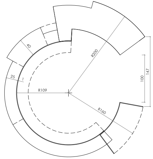
SECCIÓN H1 1:50
