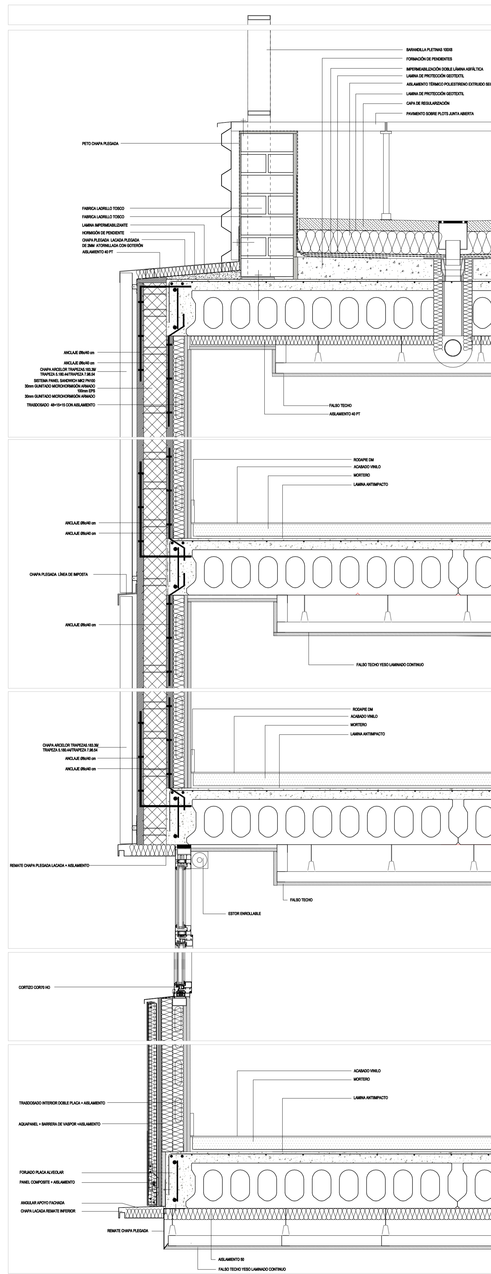
DETALLES CONSTRUCTIVOS
