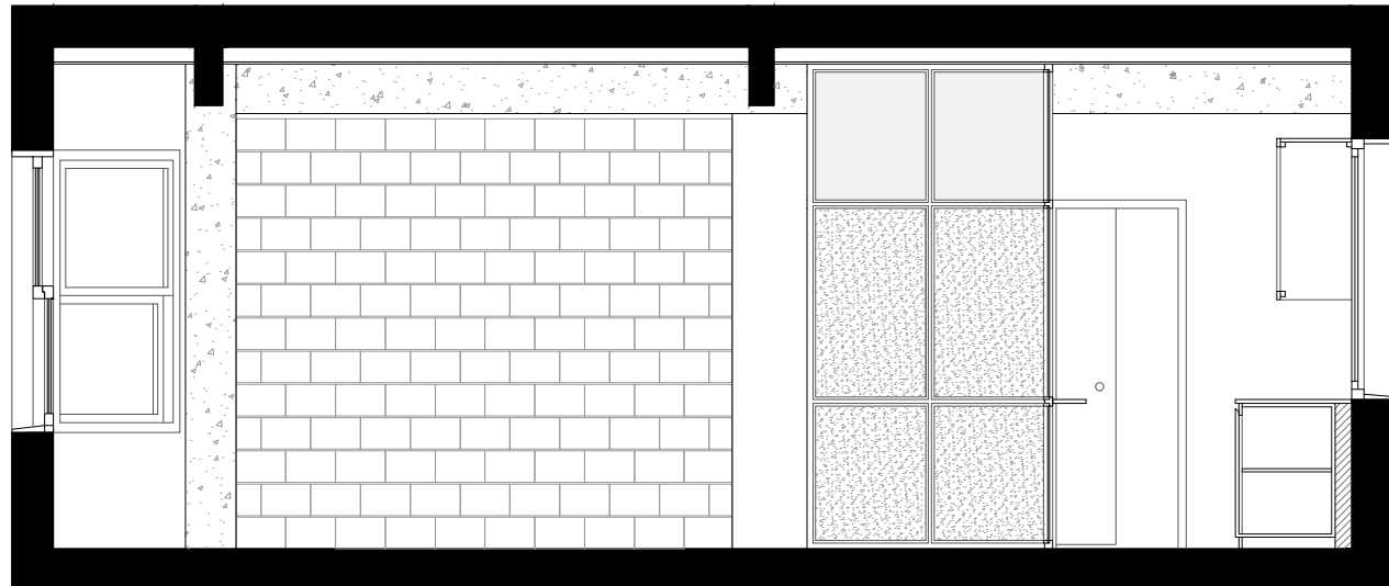
sección A-A'
