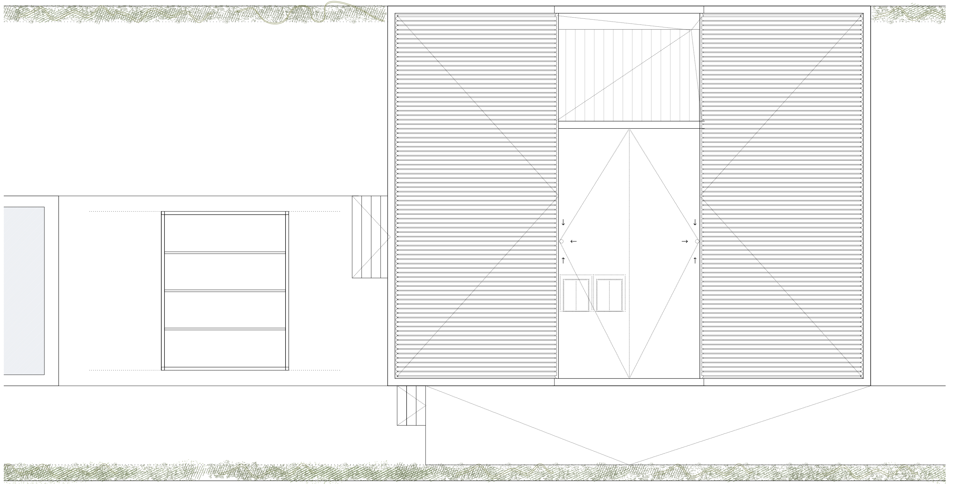
PLANTA CUBIERTA 0 0.5 1 1.5 2m
