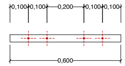
BRAZO TRANSVERSAL 40.40.3 ESC 1:20
