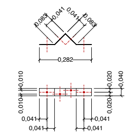
CHAPA PLEGADA 3mm ESC 1:20
