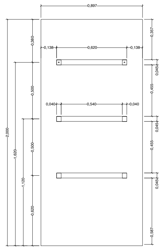
PANEL DIBOND IMPRESO EN 3mm PARA PANELES INFORMATIVOS ESC 1:20
