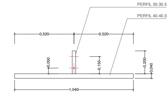
PIE EN CRUZ - ALZADO ESC 1:20
