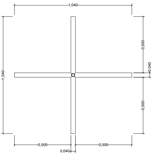
PIE EN CRUZ - PLANTA ESC 1:20
