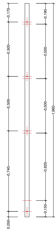
PILAR 40.40.3 ESC 1:20
