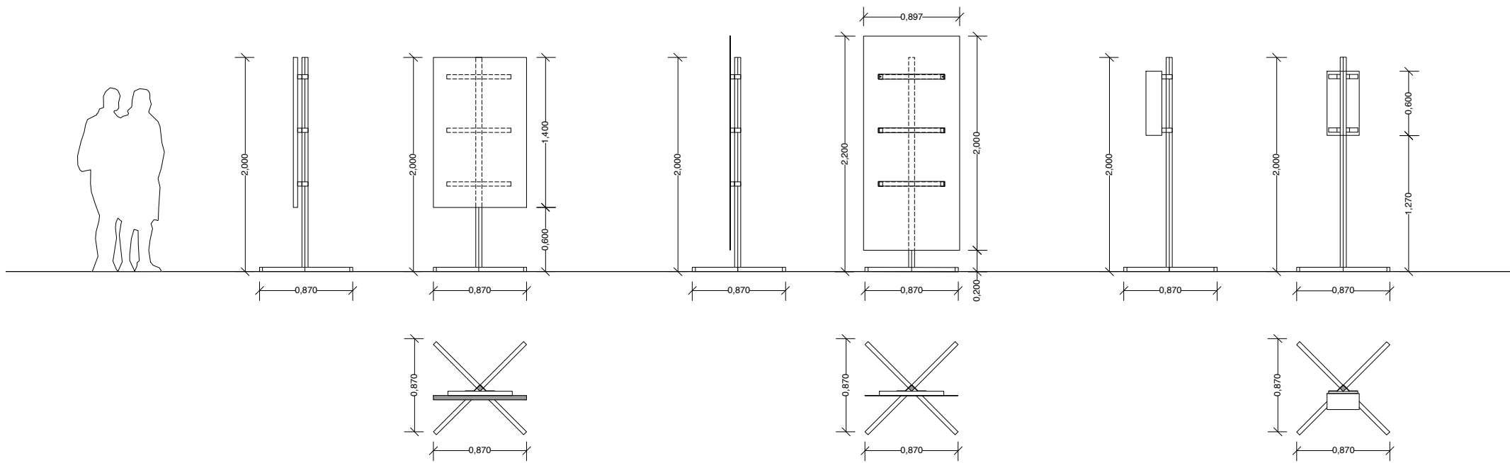
BASTIDORES PARA PANTALLAS, PANELES Y ALTAVOCES ESC. 1 /50
