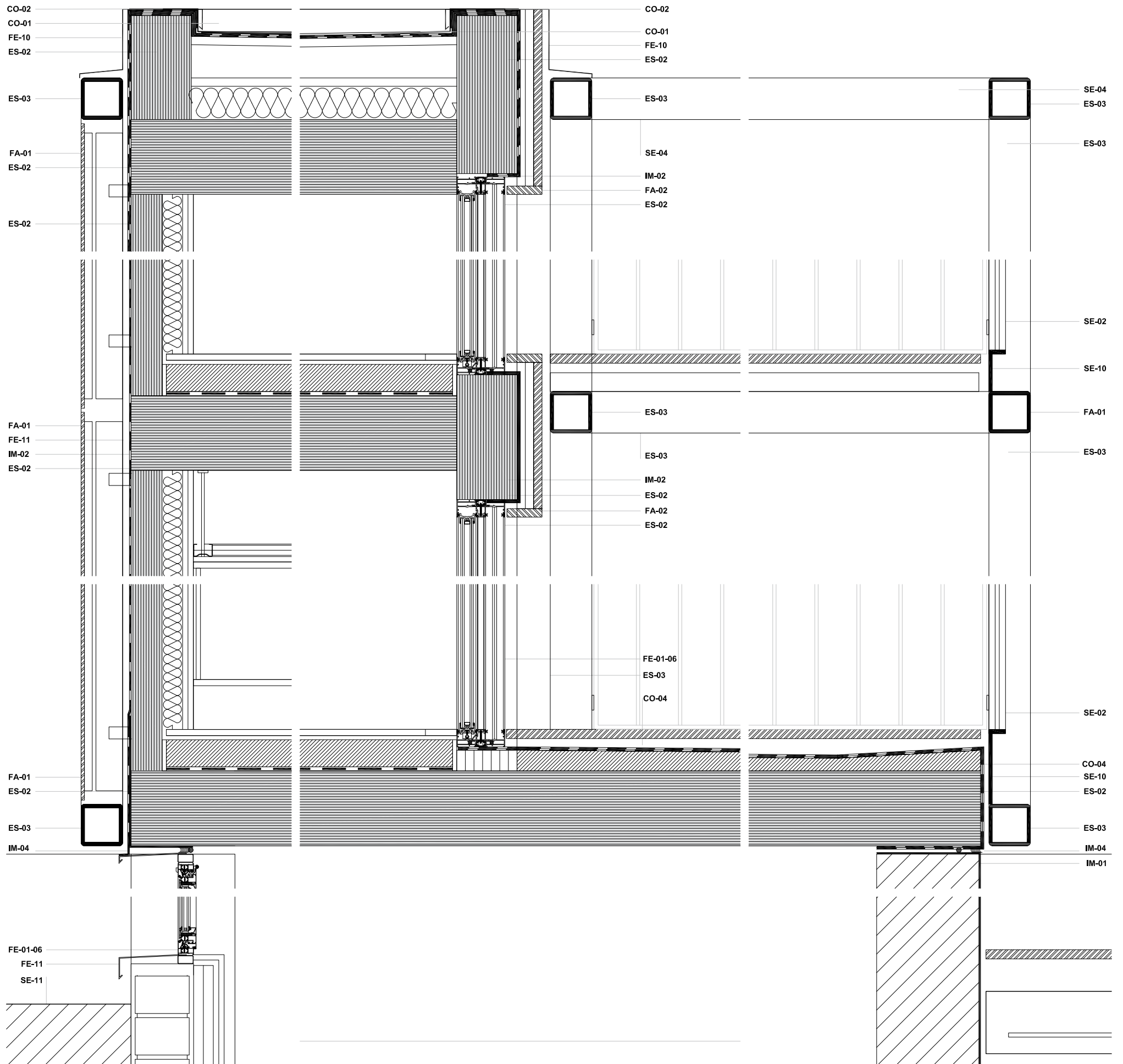
Longitudinal construction section / Sección constructiva longitudinal
