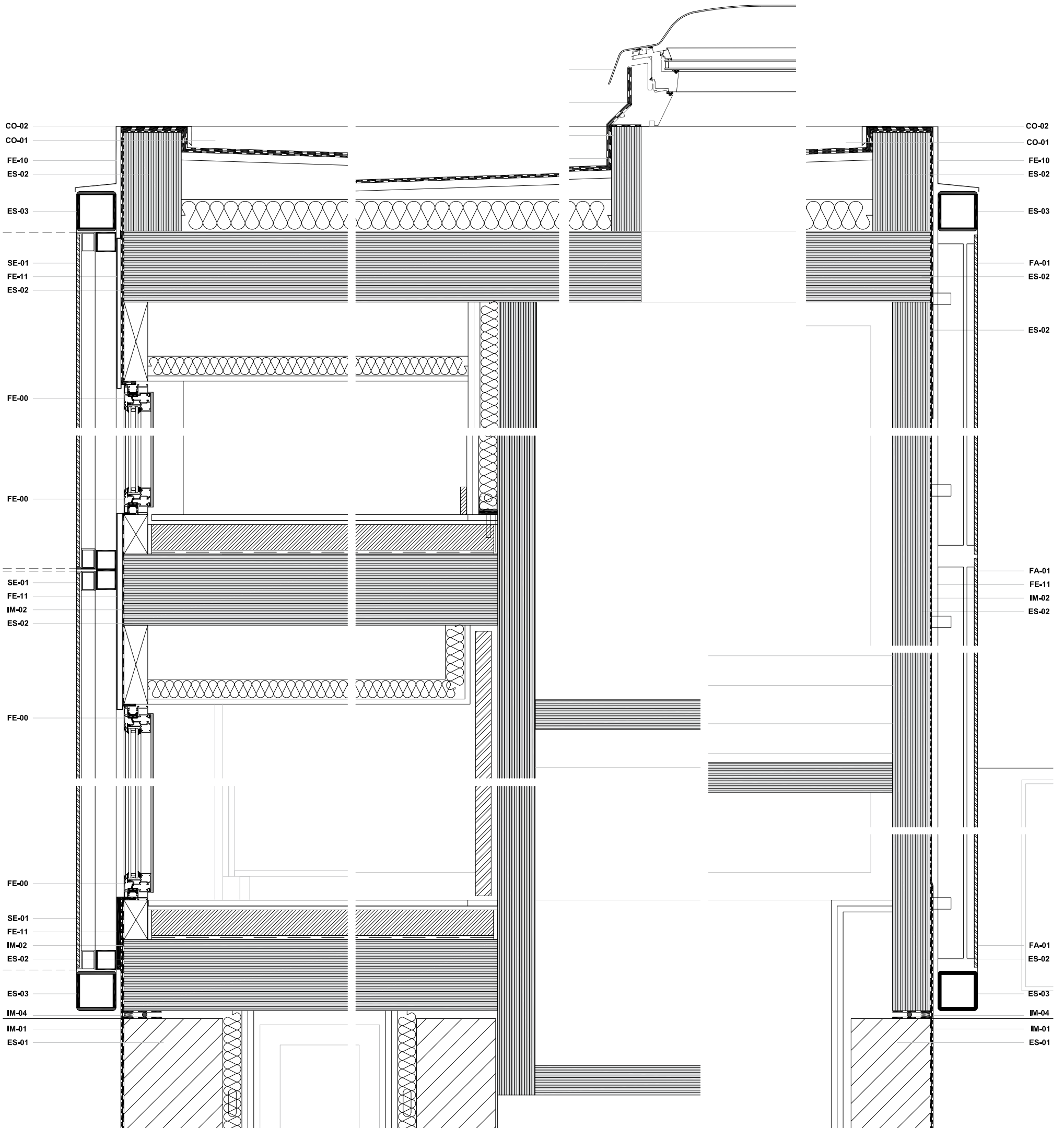
Transversal construction section / Sección constructiva transversal
