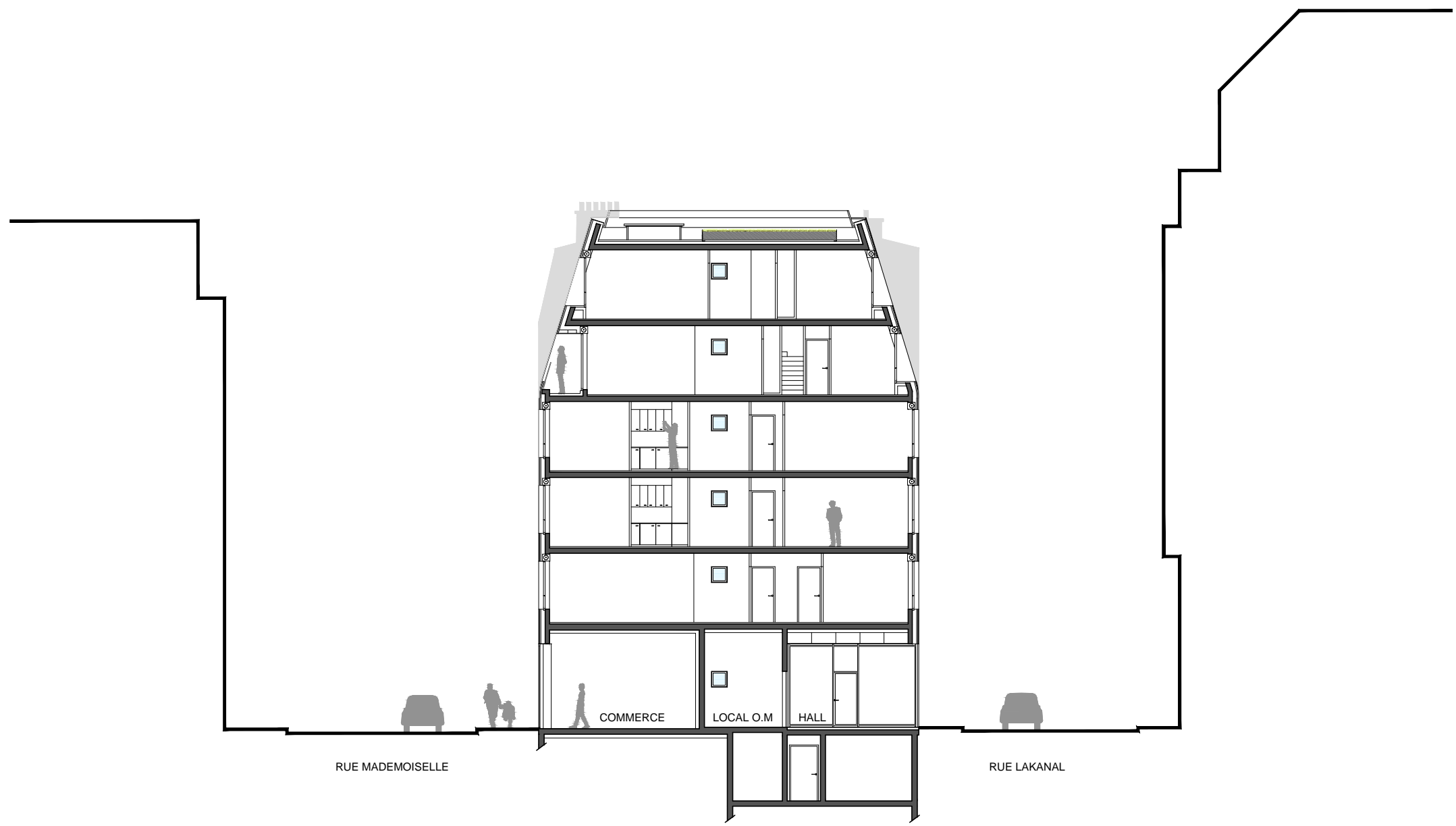
COUPE TRANSVERSALE
