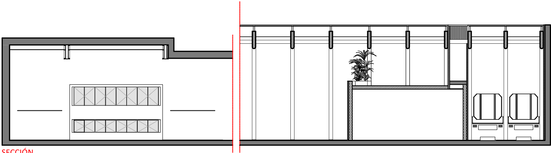
SECCIÓN DD'
