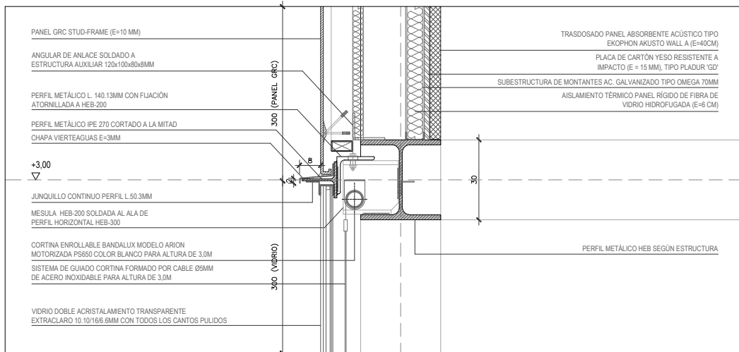
DETALLE ENCUESTRO PANEL GRC-VIDRIO
