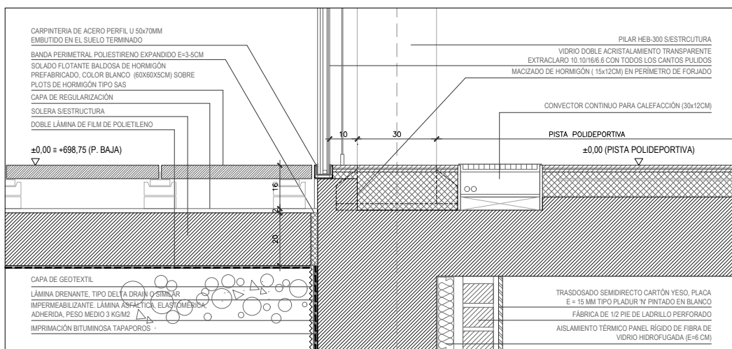
DETALLE ARRANQUE VIDRIO
