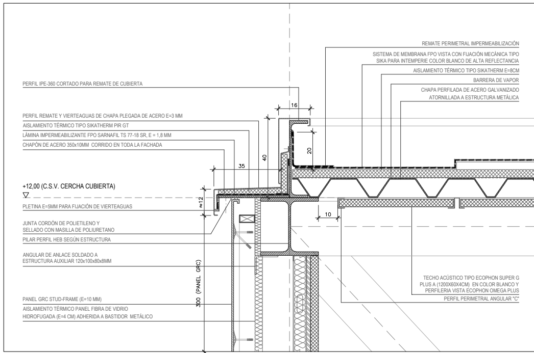
DETALLE REMATE CORNISA CON PANEL GRC
