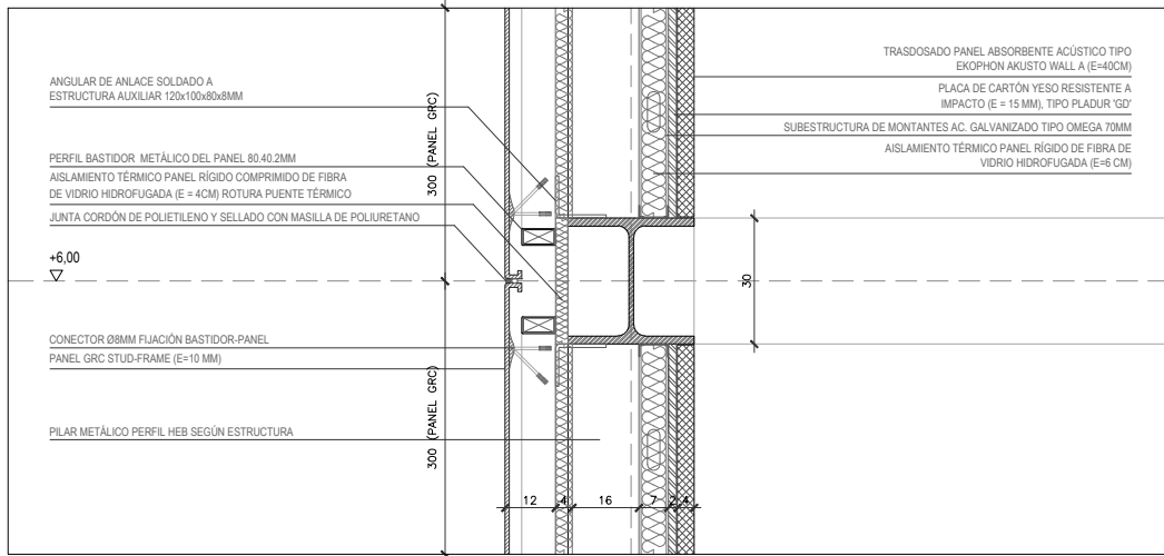
DETALLE ENCUESTRO PANEL GRC-PANEL GRC
