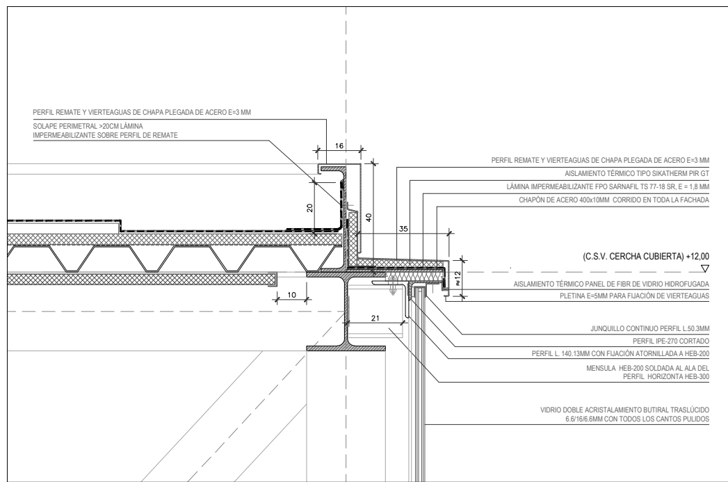
DETALLE REMATE CORNISA CON VIDRIO
