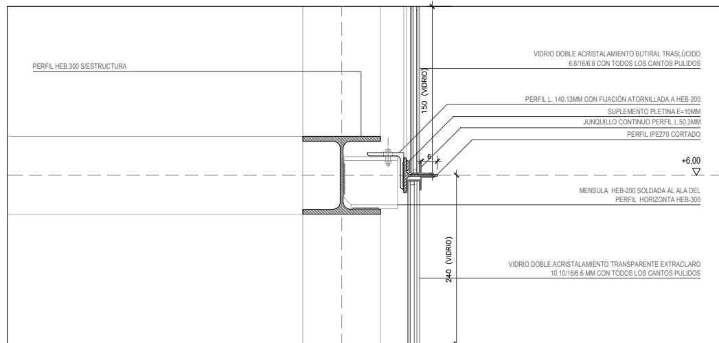
DETALLE ENCUENTRO VIDRIO-VIDRIO
