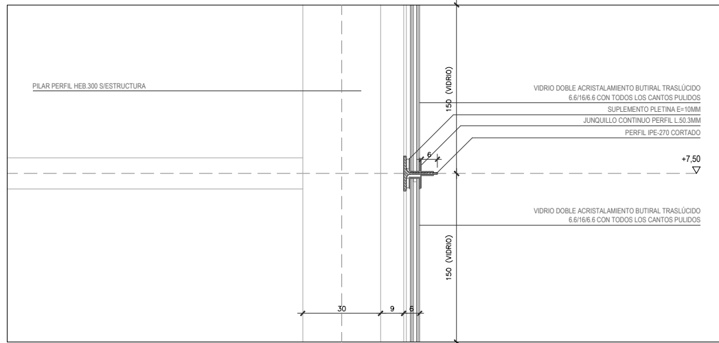
DETALLE VIDRIO MONTANTE INTERMEDIO
