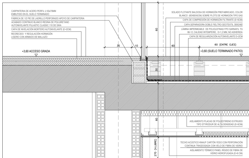
DETALLE ARRANQUE VIDRIO PATIO ALTO
