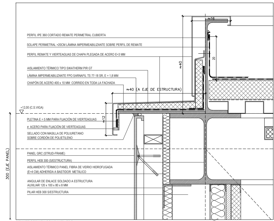
REMATE CORNISA CON PANEL GRC
