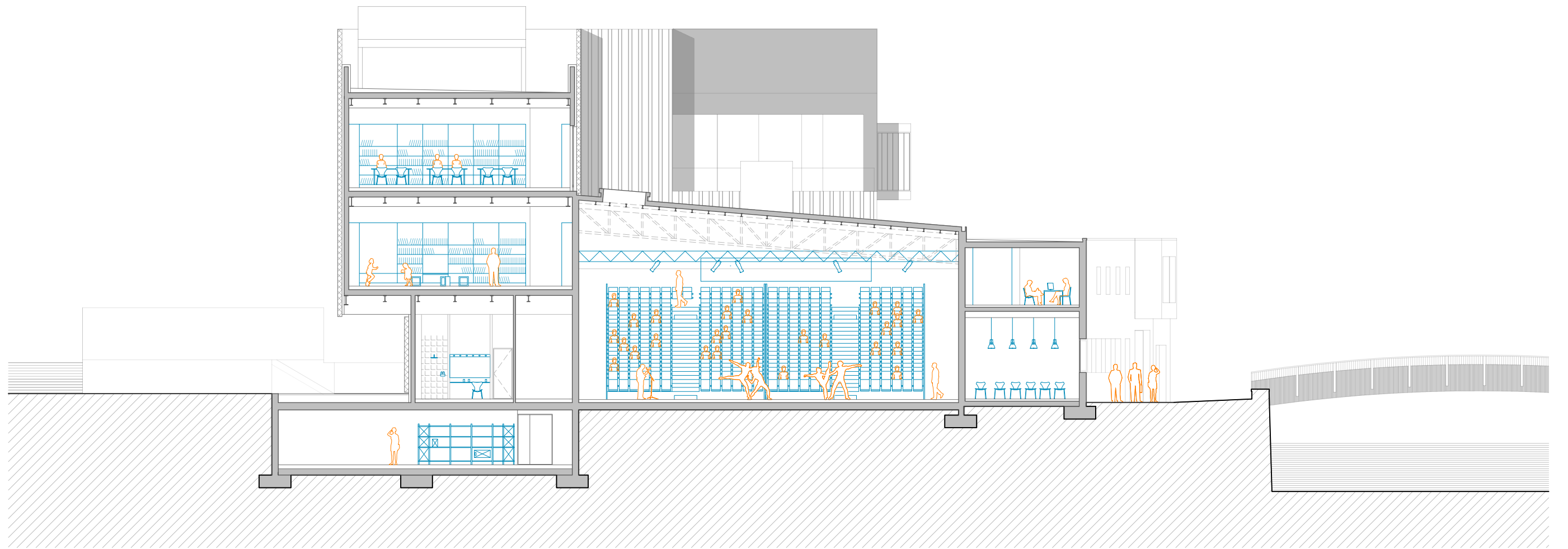
SECCIÓN TRANSVERSAL
