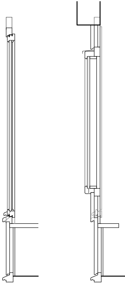
Sección AA'
