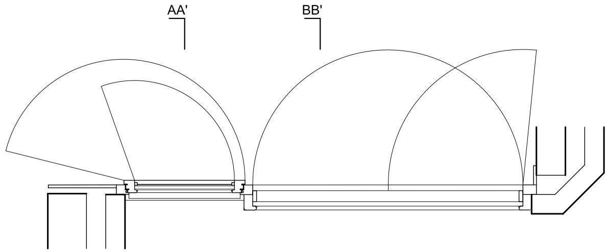
Planta
